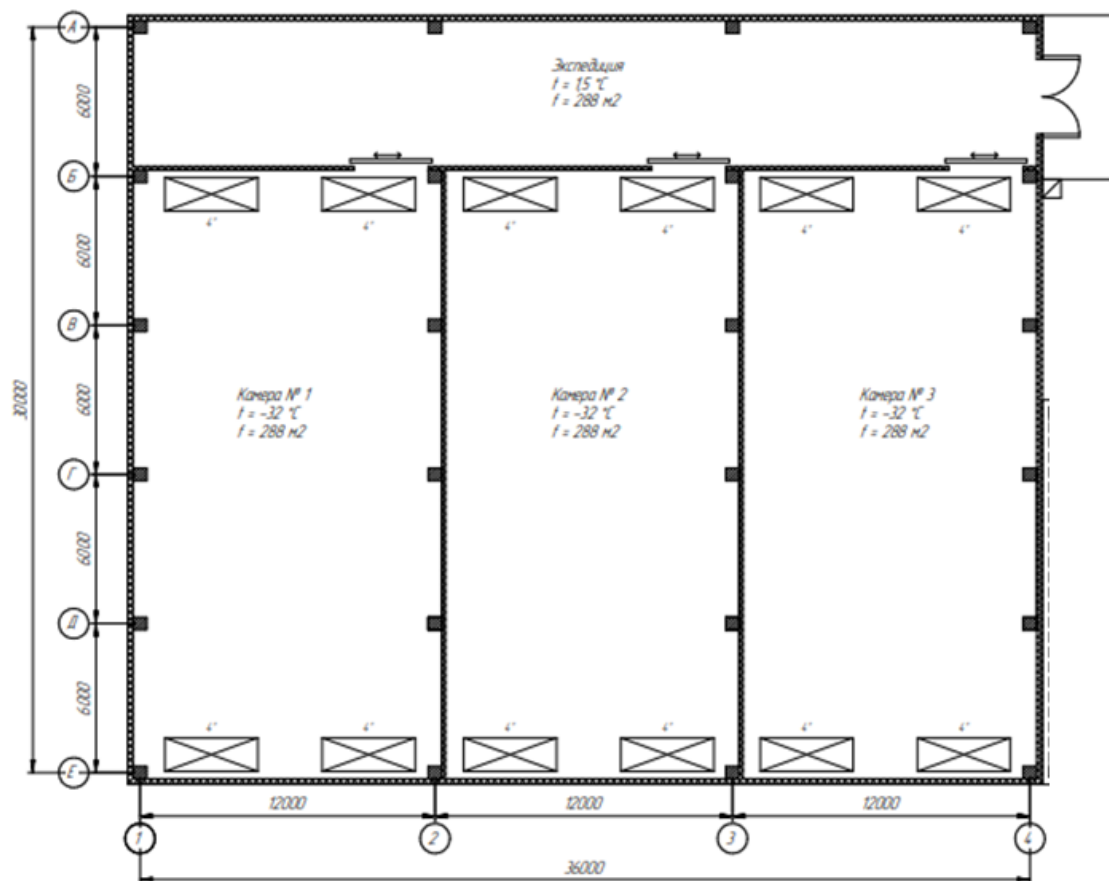
Рисунок 1 – Планировка холодильника
